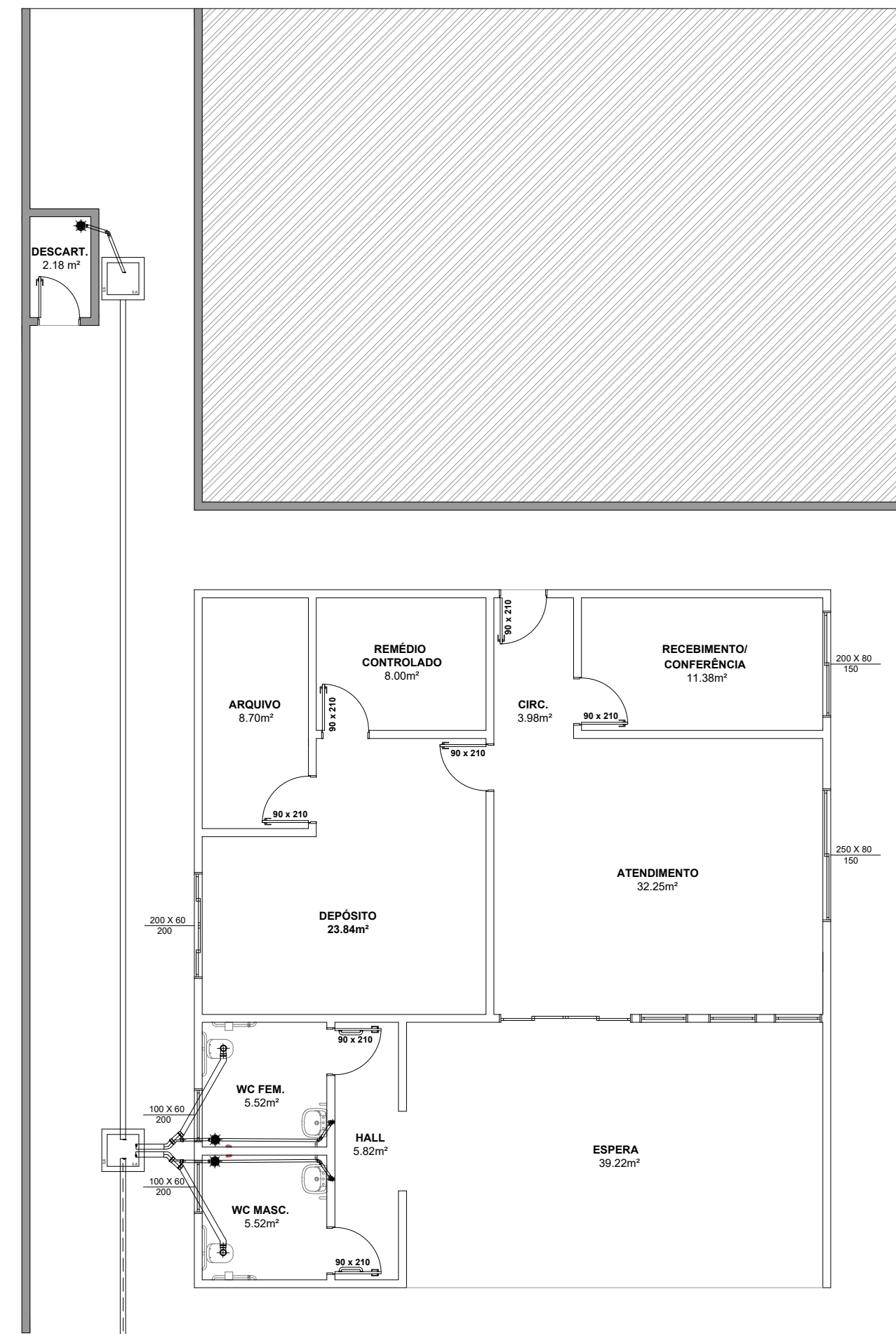
PLANTA BAIXA - ESQUEMÁTICA ESGOTO ESC.: 1/100
