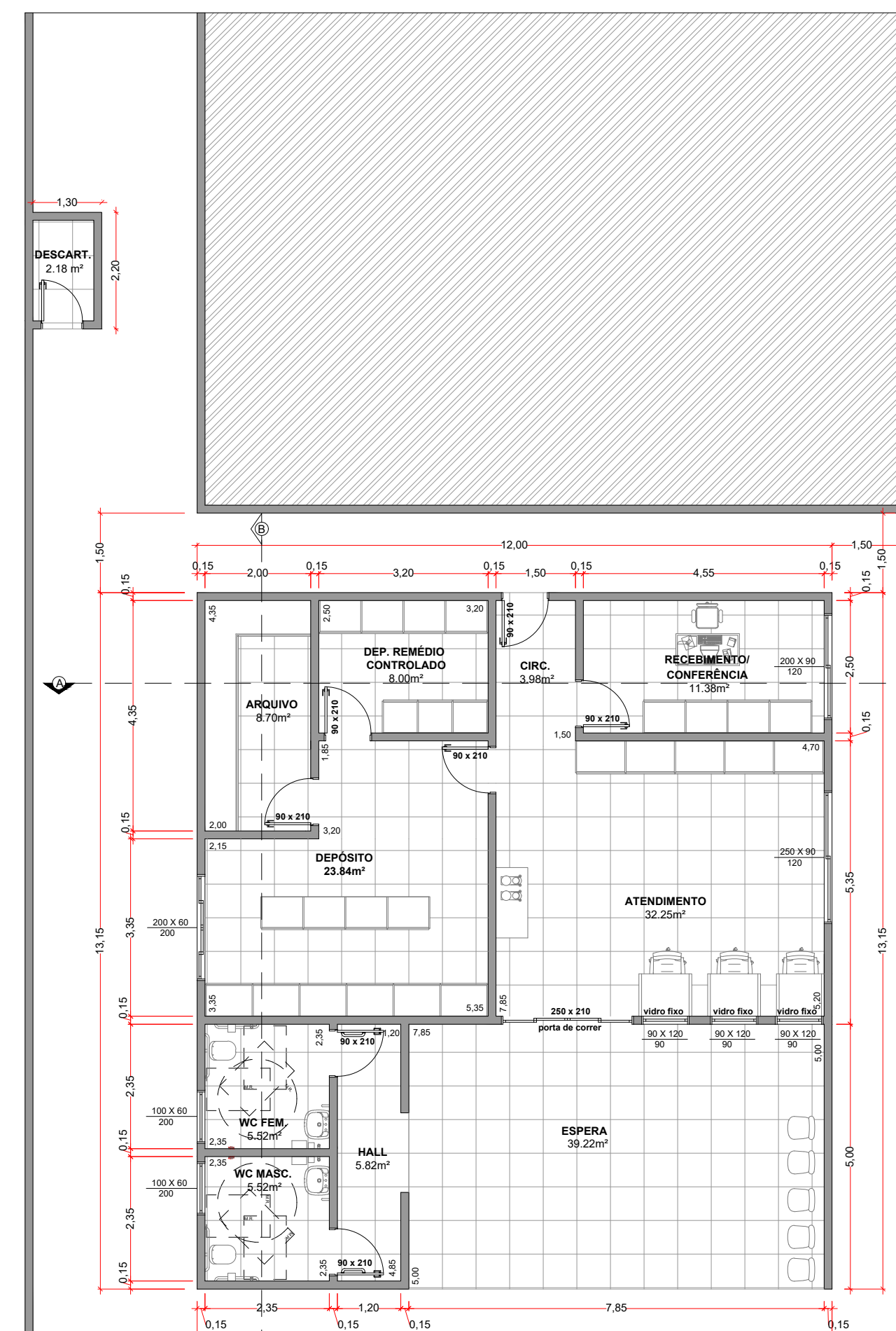
PLANTA BAIXA - LAYOUT ESC.: 1/100
