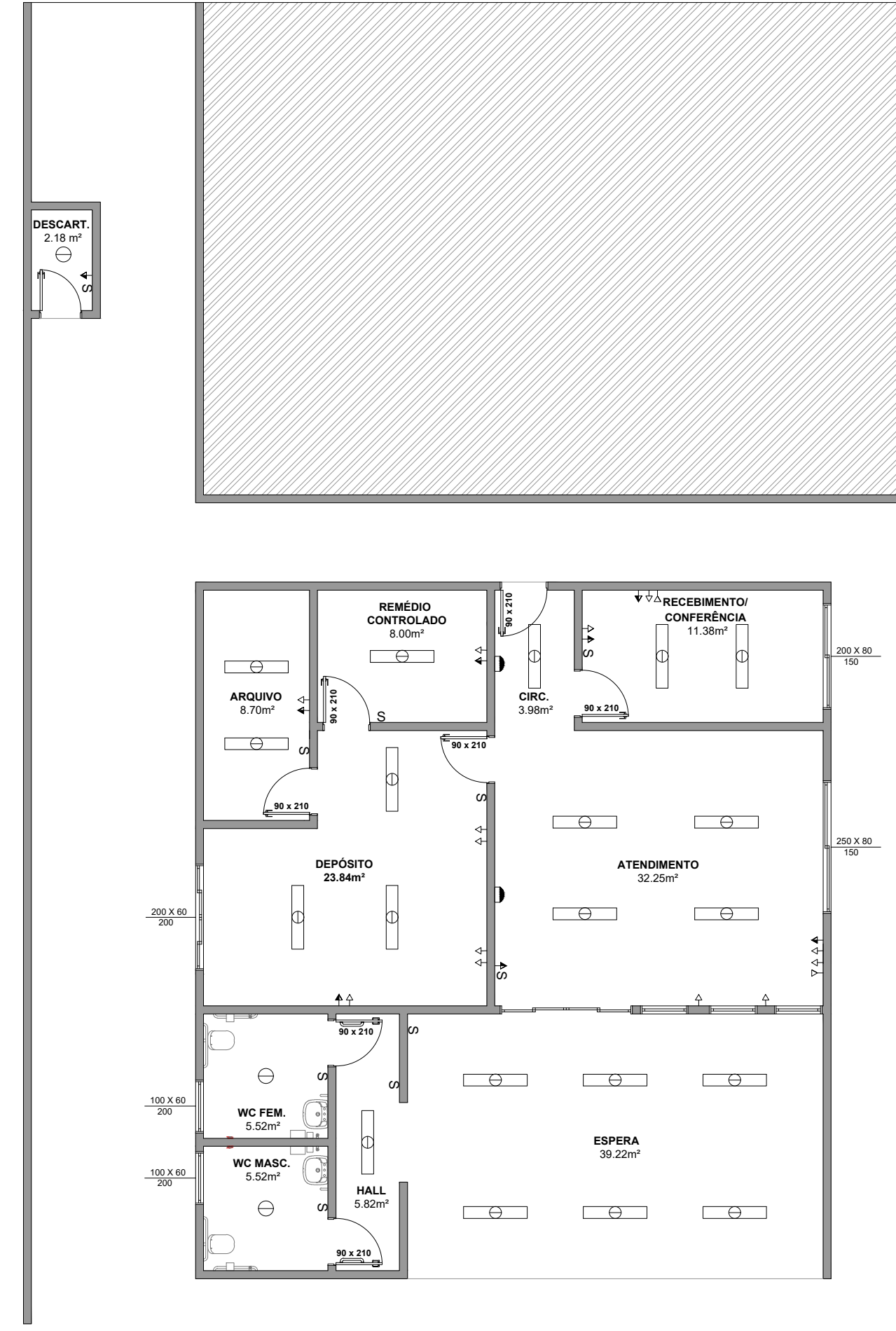
PLANTA BAIXA - ESQUEMÁTICA ELÉTRICA ESC.: 1/100
